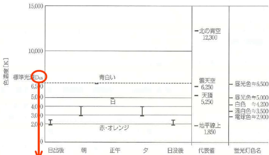
図4.11 昼光光源の色温度変化と蛍光灯色名
